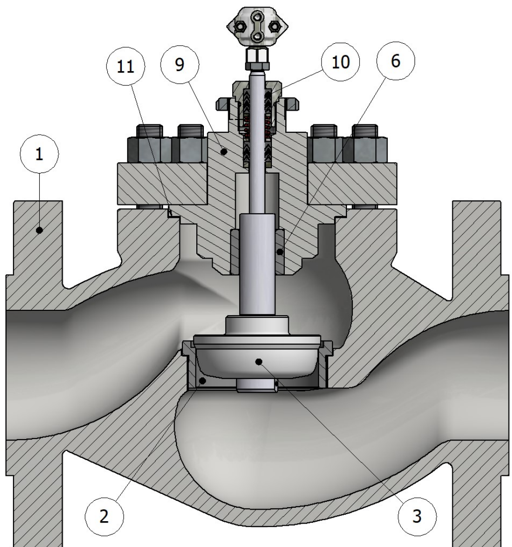
STANDARDVENTIL
